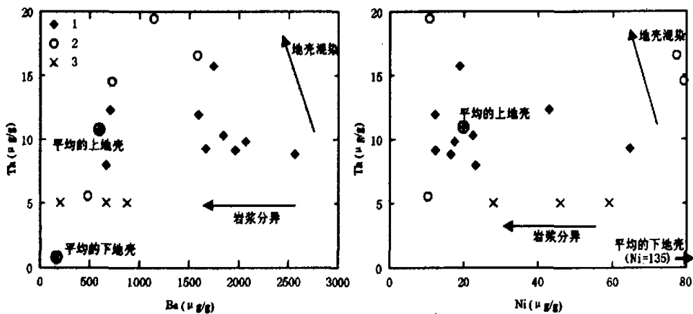
图5 安基山岩体中酸性岩石的 Ba-Th 和 Ni-Th 图解
