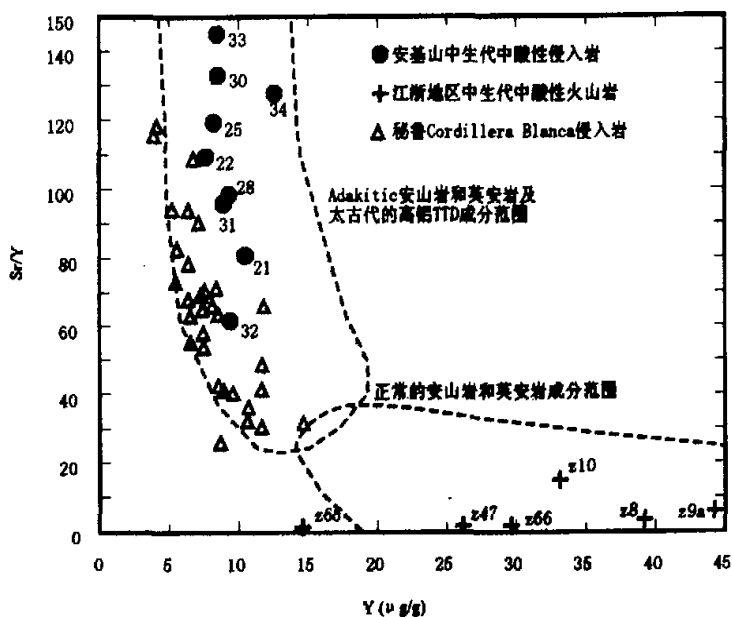
图4 安基山侵入岩的 Sr/Y-Y 成分变异图
