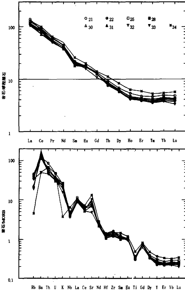
图2 安基山岩体中酸性侵入岩稀土和不相容微量元素模式
