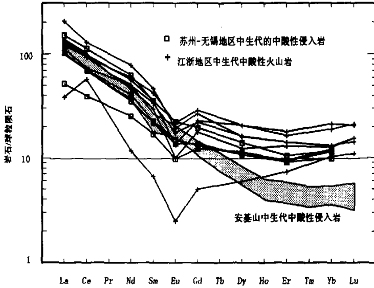
图3 安基山岩体与不具有 adakite 成分特征的中酸性火成岩稀土组成的比较
